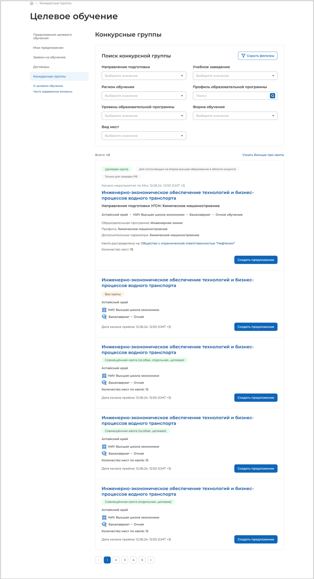
Рисунок 43 – Результат поиска
