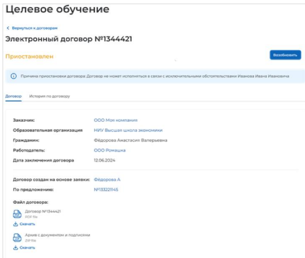
Рисунок 123 – Вкладка «Договор»
