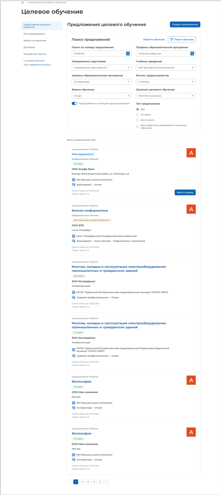
Рисунок 48 – Результат поиска
